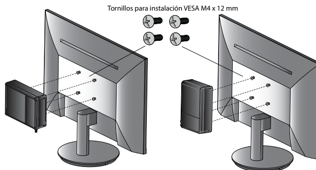
Figure 9. Instalación con Soporte VESA
