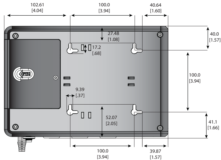
Figure 11. BC850RNC(AG-0761) Dimensions des trous de montage mural
